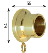
Rosetta chiusa Ø35 con gancetti Art. MS35RC
